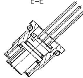
Ansicht ohne Mutter 2:1 E-E
